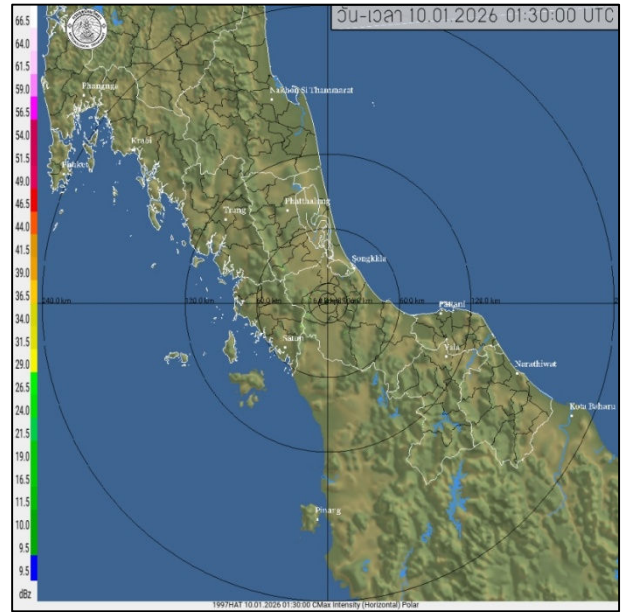
สถานีหาดใหญ่ เวลา ๐๘.๓๐ น.
