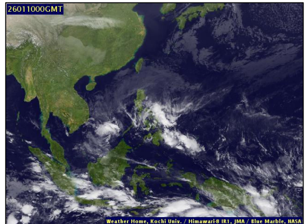
ภาพถ่ายดาวเทียม วันที่ ๑๐ ม.ค. ๒๕๖๙ เวลา ๐๗.๐๐ น.
