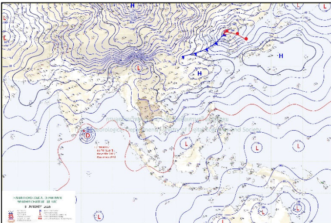
แผนที่อากาศ วันที่ ๑๐ ม.ค. ๒๕๖๙ เวลา ๐๑.๐๐ น.
